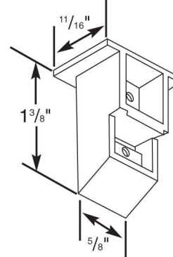
24210 - Top Sash Guide
