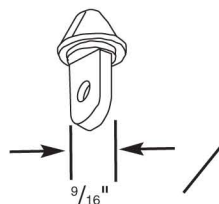
24340 - Balance Cap
