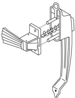
42230 - Black Storm Door Latchset
