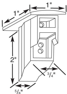
28340 - Top Sash Guide
