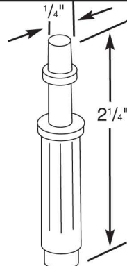
Top Pivot
