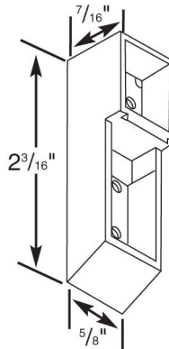
25500 - Top Sash Guide
