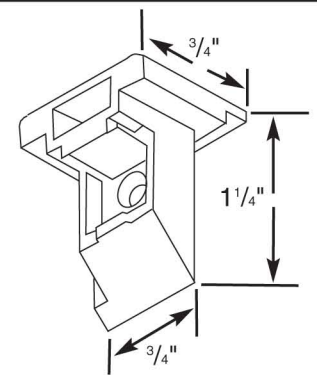
28800 - Top Sash Guide (Pair)
