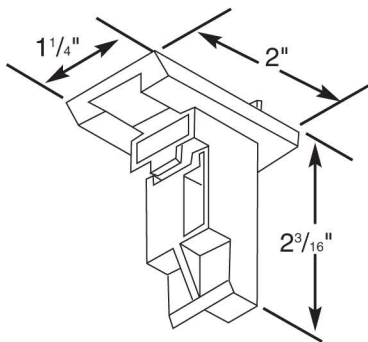
25620 - Top Sash Guides (Pair)
