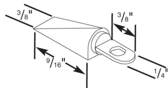
24150 - Balance Cap
