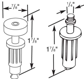
Top Pivot & Guide Wheel
