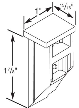
25550 - Top Sash Guide
