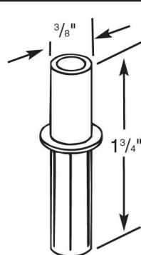
Top Pivot
