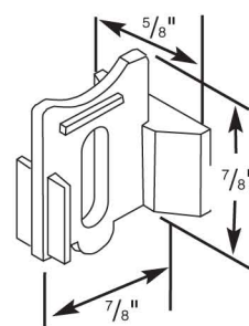
24170 - Top Sash Guide
