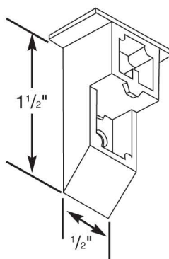
24190 - Top Sash Guide
