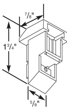
24160 - Top Sash Guide
