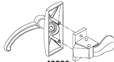
42520 Lever storm door Lockset
