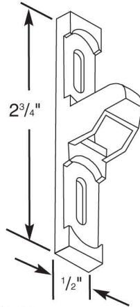
12060 - Patio Door Keeper
