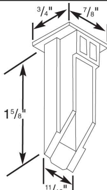
24780 - Top Sash Guide
