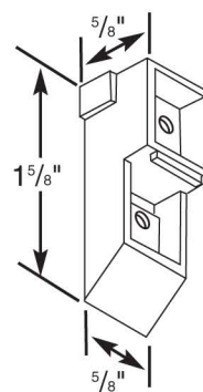
28030 - Top Sash Guide
