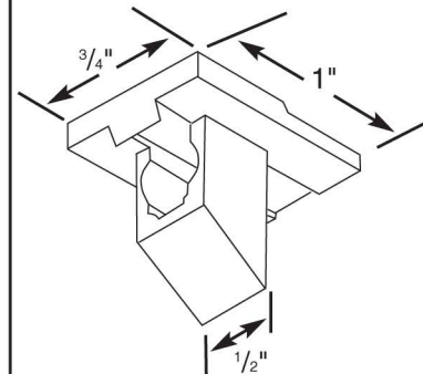
28320 - Top Sash Guide
