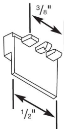
24260 - Sash Guide
