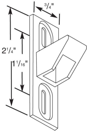
12010 - Patio Door Keeper
