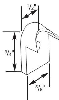
28950 - Top Sash Guide
